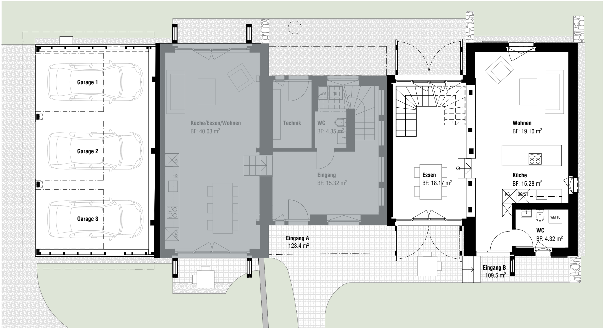
Erdgeschoss - Wohnung B Wartrain 3 in 6331 Hünenberg
